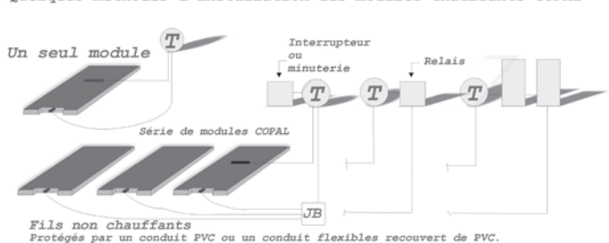
Quelques méthodes d'installation des modules chauffants COPAL
